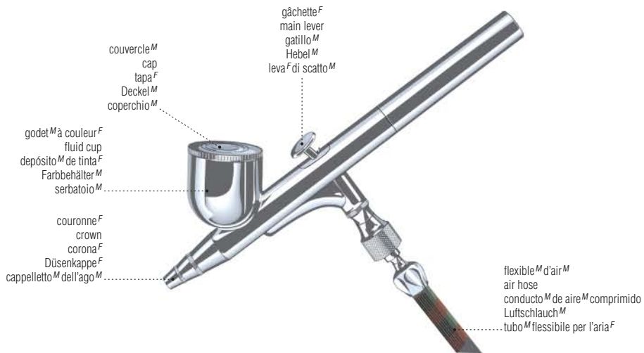
gâchette F main lever gatillo M Hebel M leva F di scatto M
